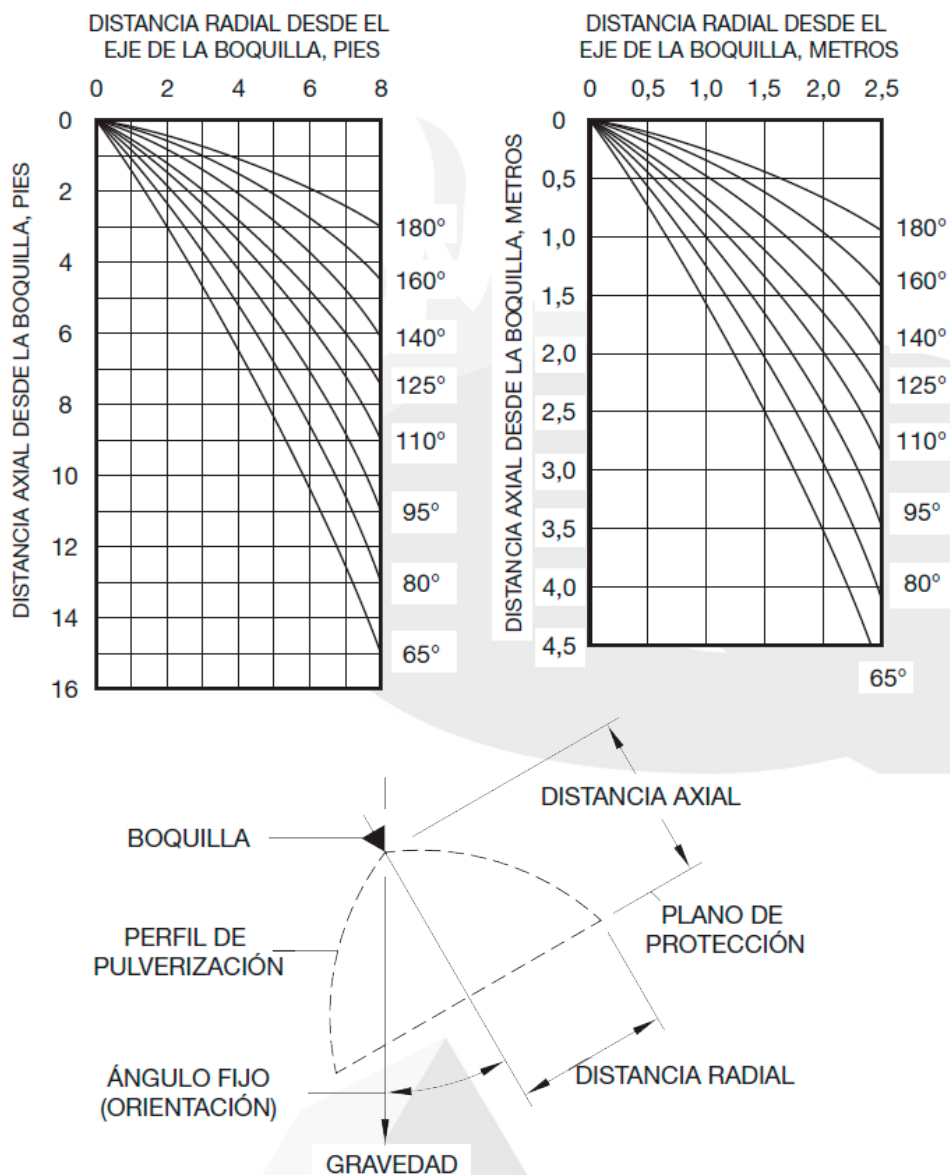
Figura2. Datos de diseño de distribución del agua.
